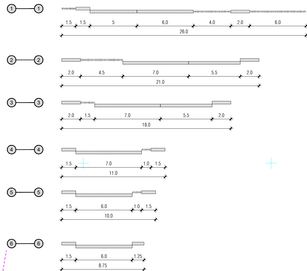
POREČNI PROFILI
