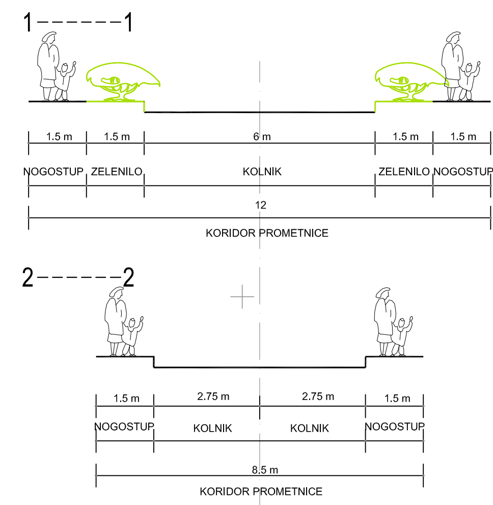
POPREČNI PROFILI PROMETNICA MJ 1:100
