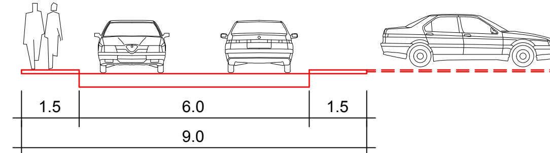
PRESJEK B-B
