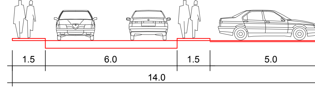
PRESJEK C-C
