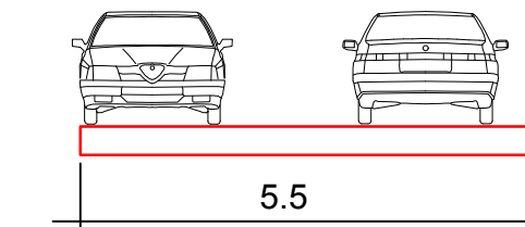
PRESJEK E-E
