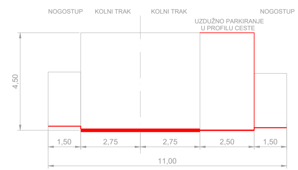
PRESJEK 2-2
