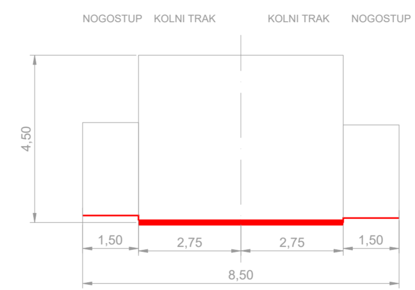
PRESJEK 2-2
