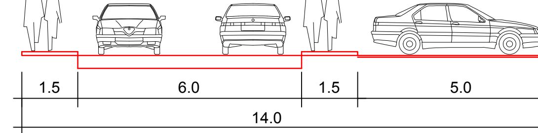
PRESJEK E-E
