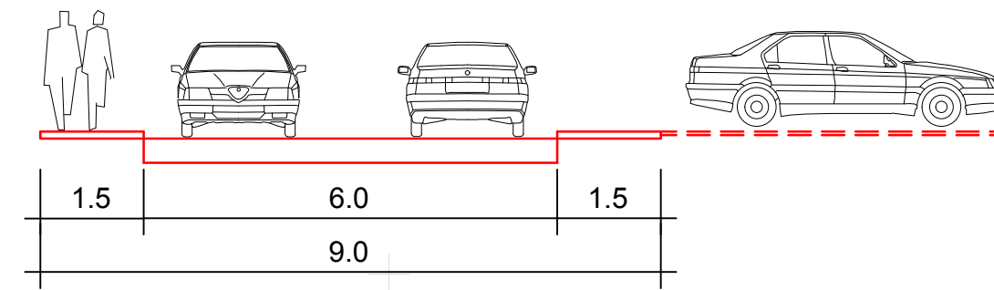
PRESJEK C-C
