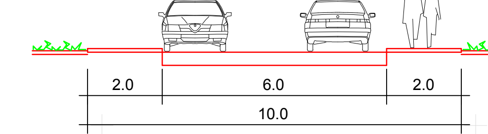
PRESJEK B-B
