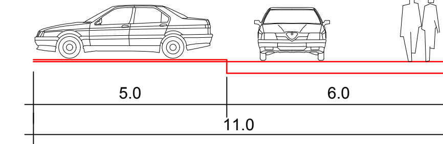
PRESJEK D-D
