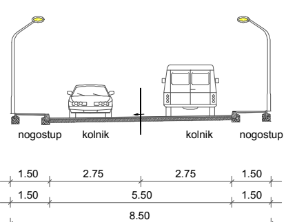
POPREČNI PRESJEK B-B ZA SABIRNU ULICU SU2 I OSTALU ULICU OU1
