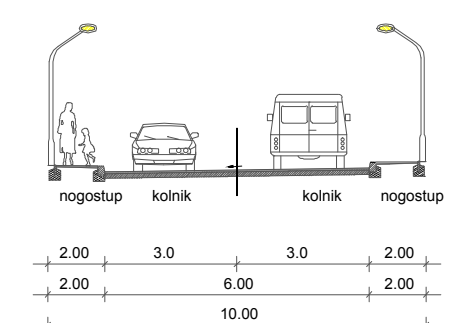
POPREČNI PRESJEK A-A ZA SABIRNU ULICU SU1
