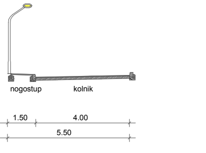
POPREČNI PRESJEK D-D ZA OSTALU ULICU OU3
