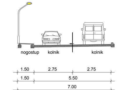
POPREČNI PRESJEK C-C ZA OSTALU ULICU OU2
